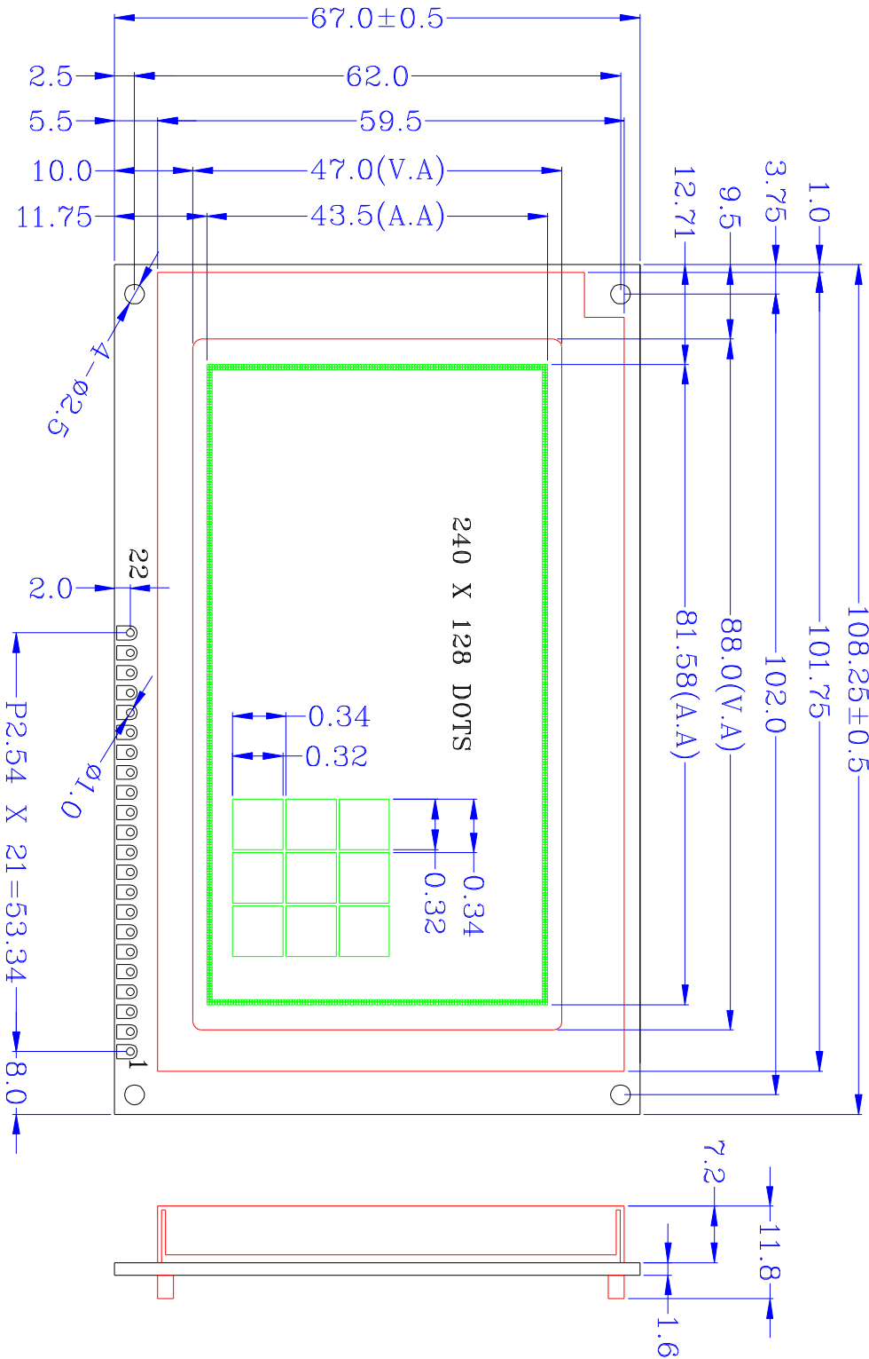
模組外形結構圖
