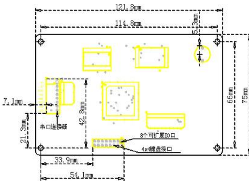
4.3 寸模块外形尺寸
