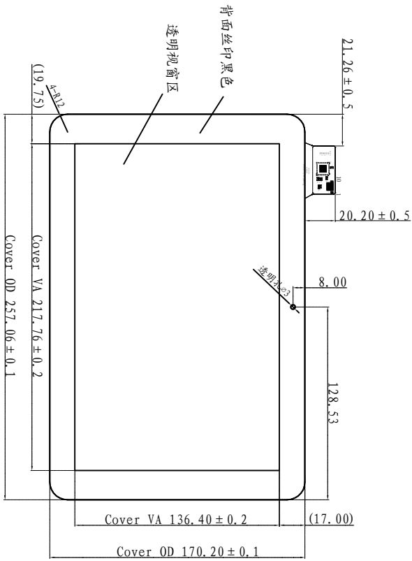
正视图
