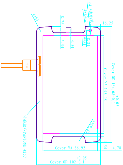
正视图
