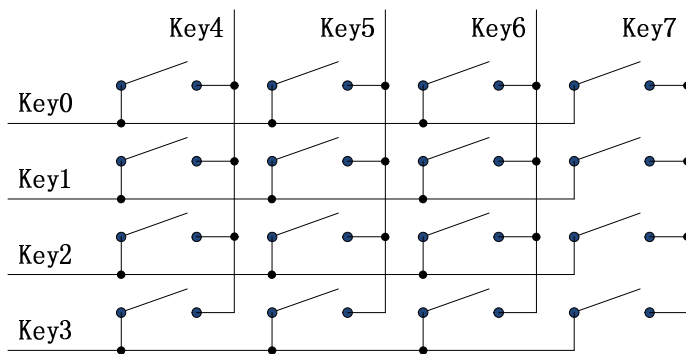
图 矩阵按键示意图
