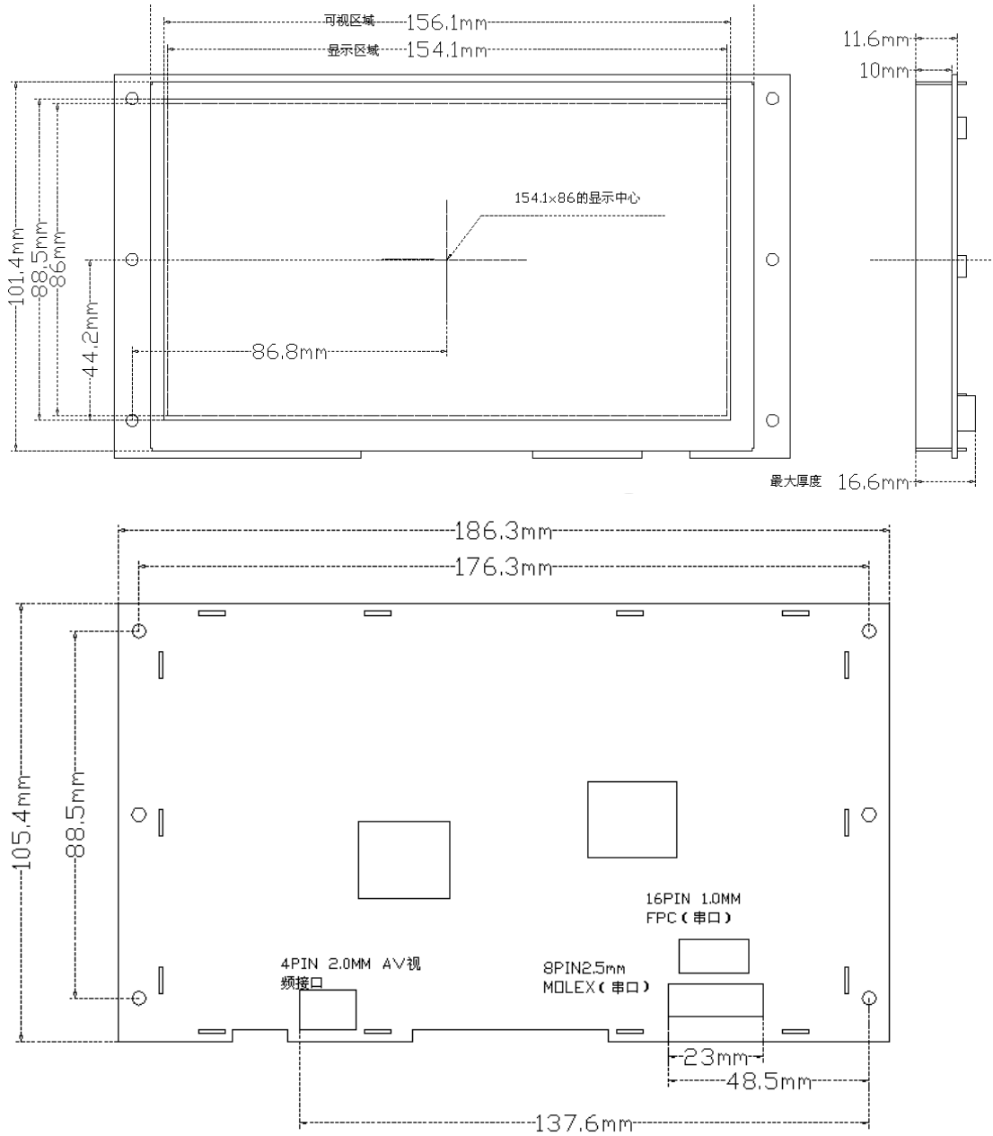
图 1 模块外形尺寸
