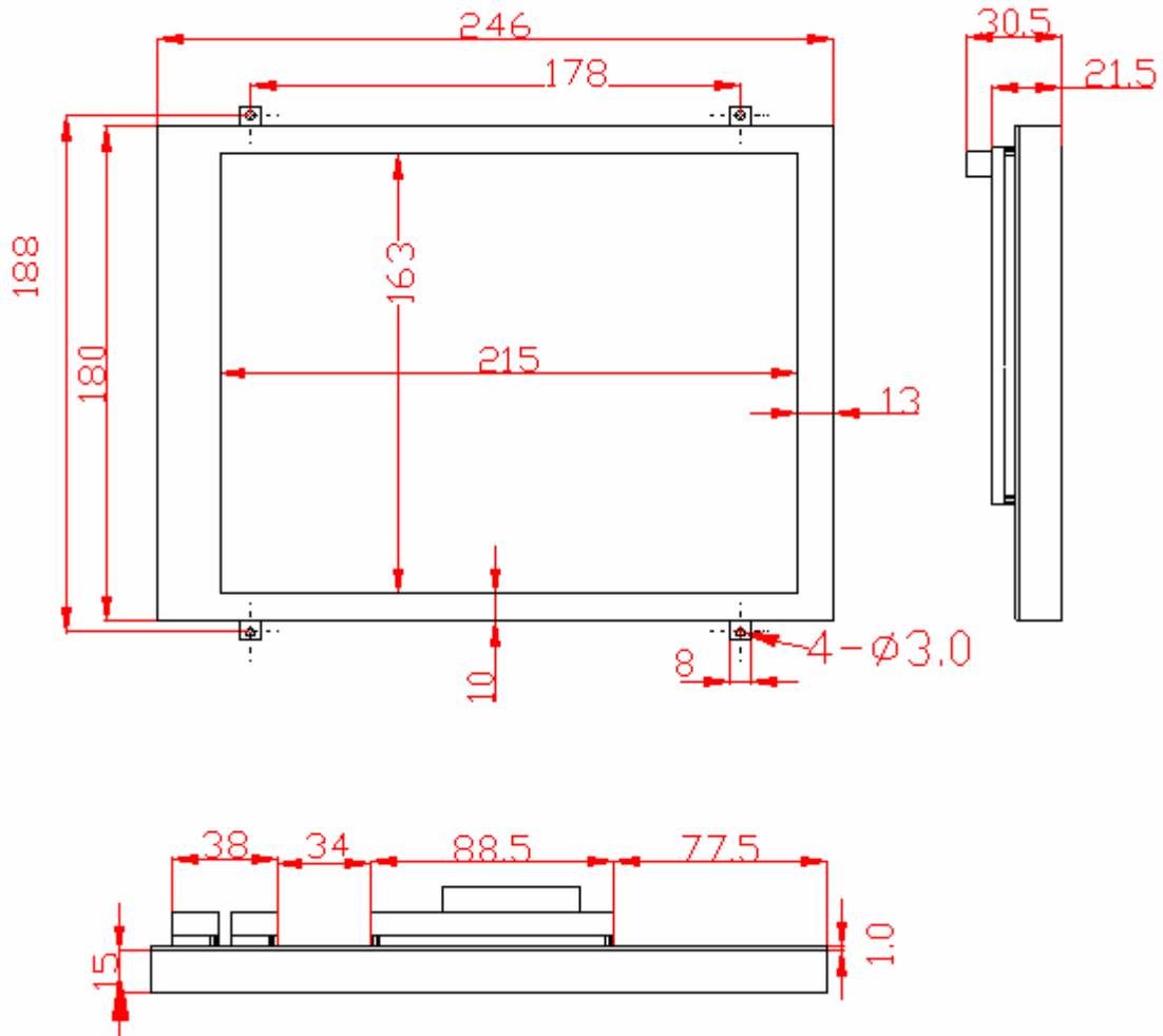
LR-104VRAM液晶显示器安装尺寸图
